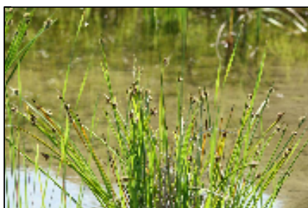
カンガレイ
